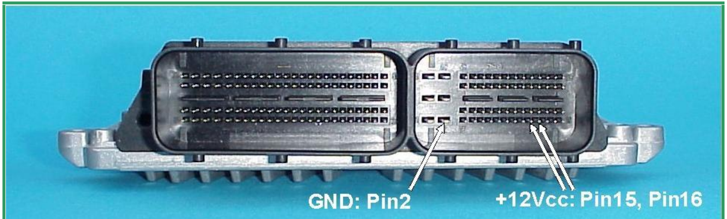
Рис. А: Разъем блока Bosch ME9.0 .
