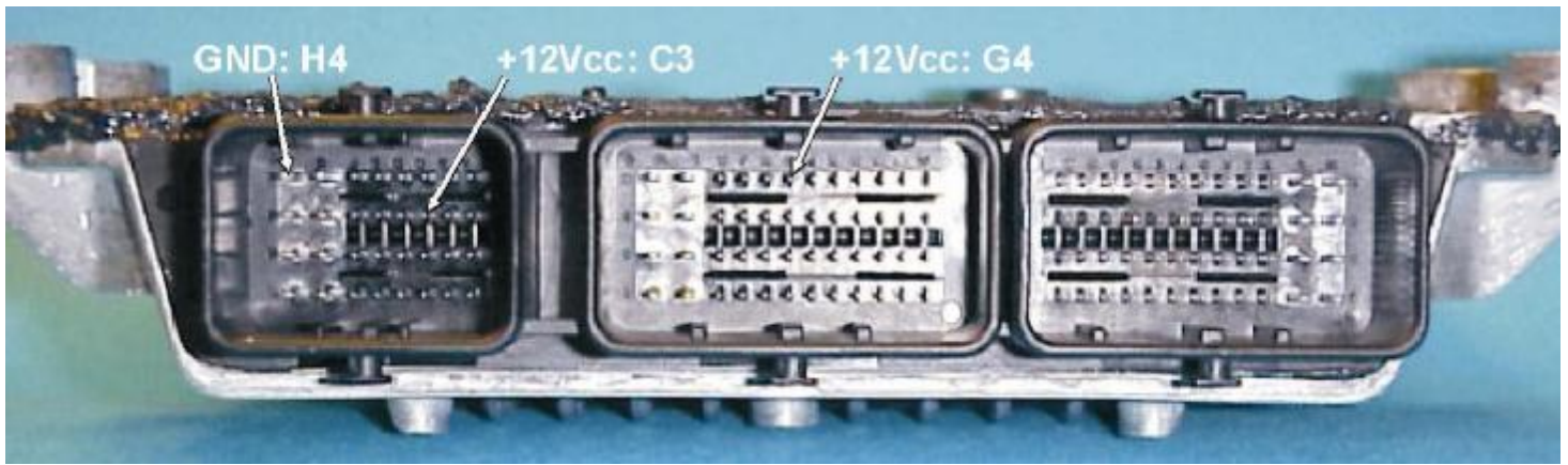
РисА: Распиновка для подключения питания блоков SID202 а так же блоков Siemens SID803(A) . Эта инструкция для блоков SID202 Так же справедлива и для SID803A.
