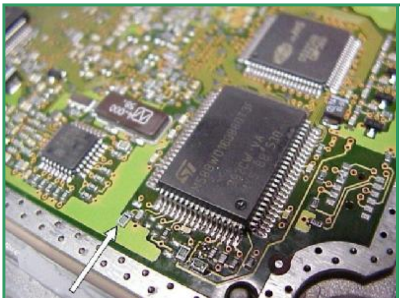
Рис.С: На этом Marelli MJD (с другим дизайном) резистор уже выпаян.
