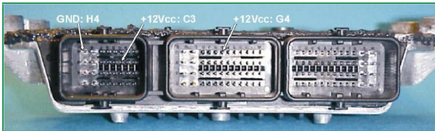
Рис.А: Распиновка по питанию для блоков Siemens SID206 ECU аналогично блоку Siemens SID803
