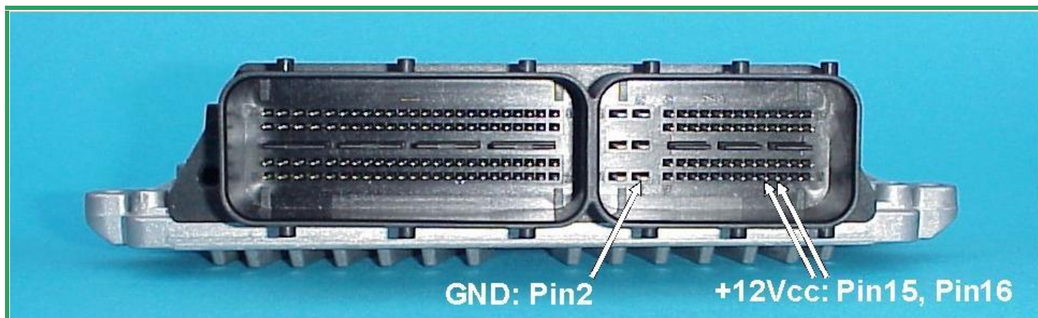
Рис. А: Разъем блока Bosch MED9.7
