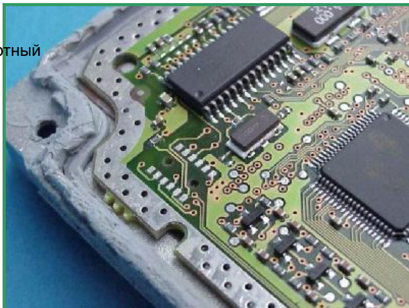
Рис. D: Площадка BDM в блоках управления Marelli
