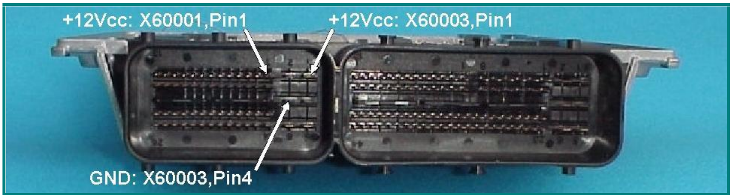
Рис. А Разъем блока управления Siemens MSV70 (аналогичен блоку MSS65 ).
