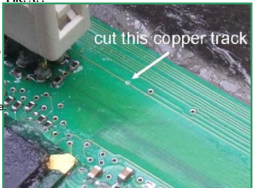
Рис.В Указанная дорожка должна быть «разорвана»
